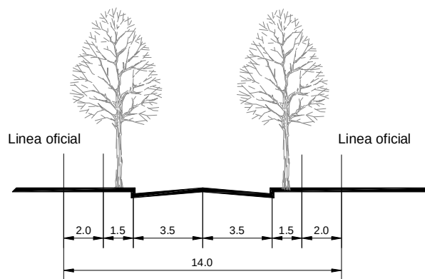
P4 PERFILES DE CALLES DE 14M
